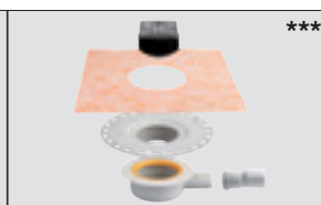
KERDI-DRAIN-BASE 1 Set (con diseño de rejilla 1)
